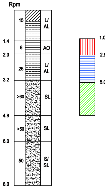
Malagnino (4 prove statiche) (Centro ricreativo)
