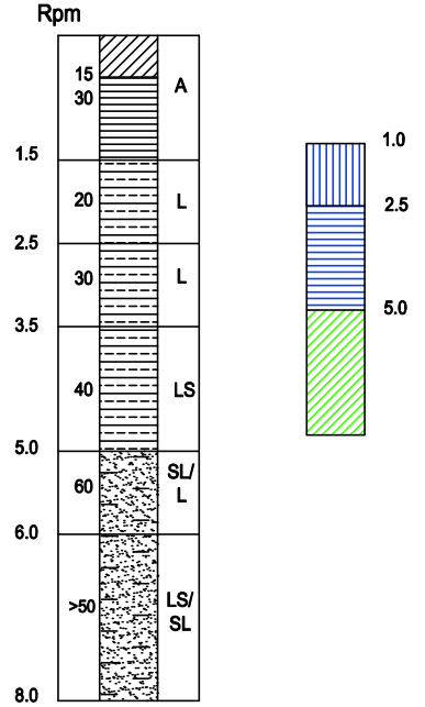
S. Giacomo di Lovara (6 prove statiche)
