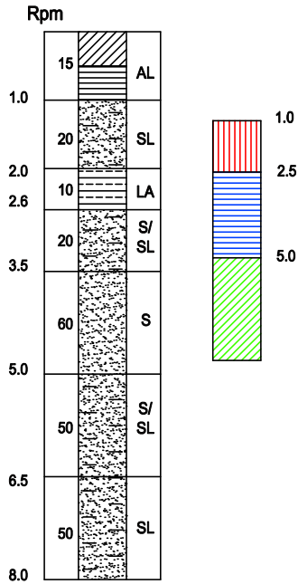
Malagnino (2 prove statiche) (Tribunetta Campo sportivo)
